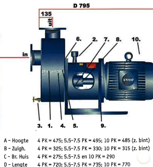
Maatschets en onderdelenlijst Goan type DA • 4-, 5.5-, 7.5- en 10 PK
