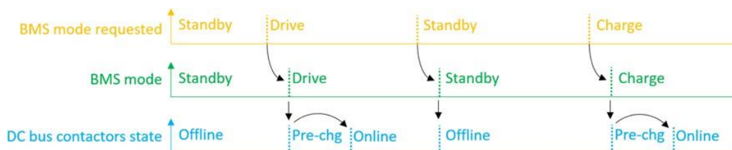
Afbeelding 33 Volgorde STAND-BY / DRIVE / CHARGE / ALTERNATIEVE LADING
