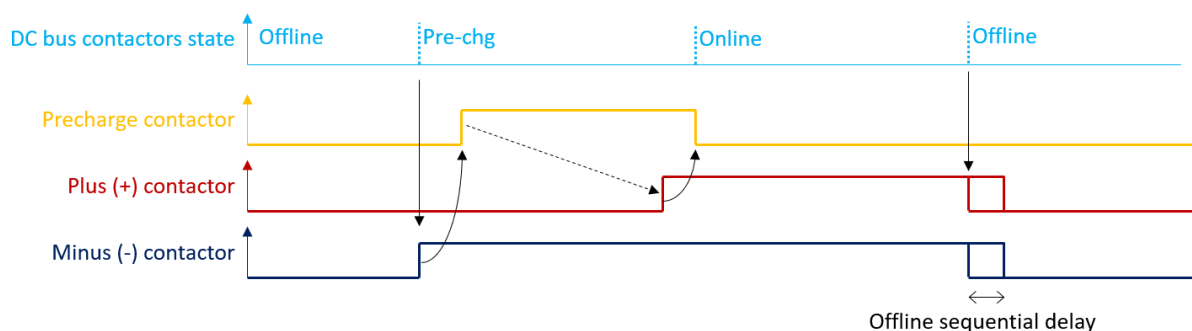
Figuur 55 Voorlaadprocedure HVDC-bus
