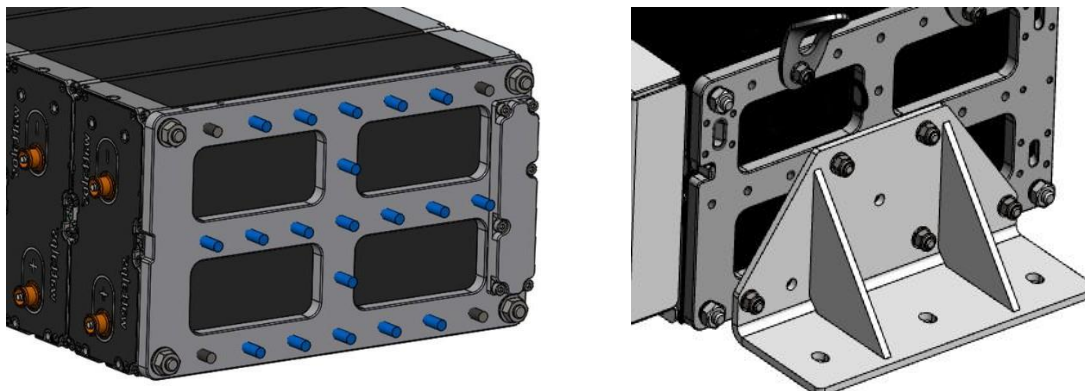
Afbeelding 11: Gedetailleerd overzicht van de bevestigingspunten
