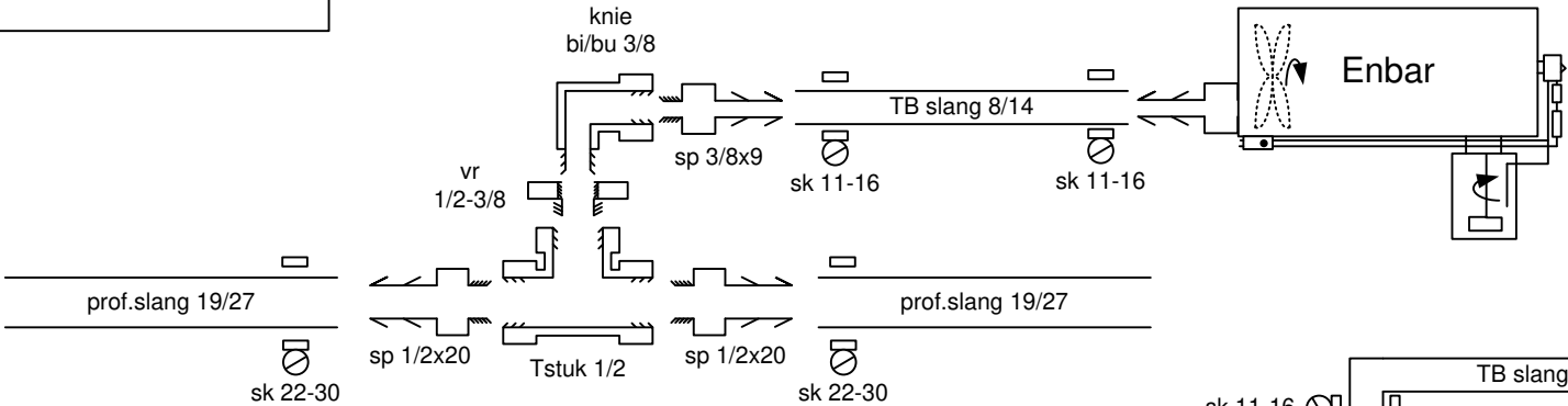
Aftakking enkele Enbar
