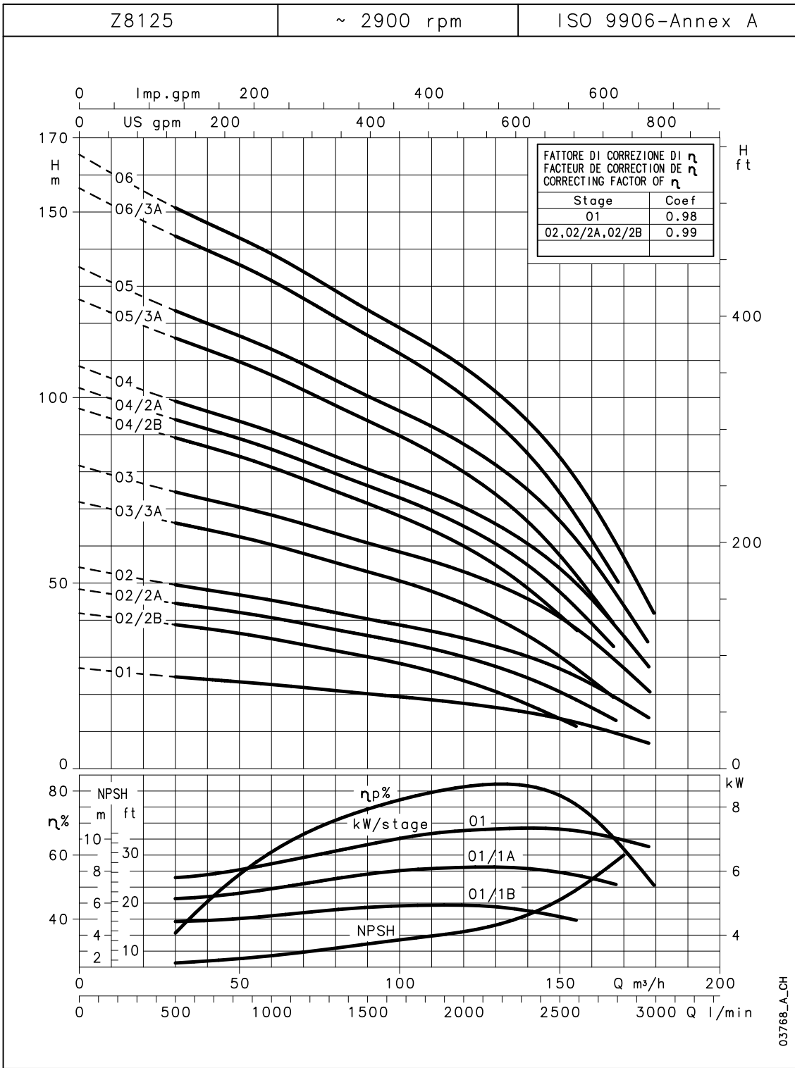
Capaciteitengrafiek Z8125 serie 1-6 waaiers bij 50 Hz, 2-polig
