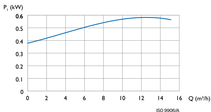
Vermogensgrafiek Grindex Micro 50 Hz
