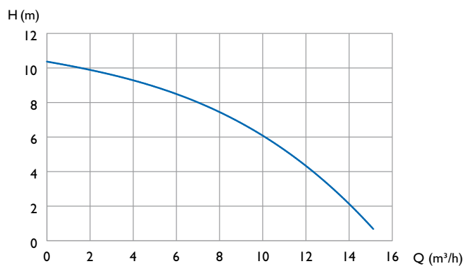
Capaciteitsgrafiek Grindex Micro 50 Hz
