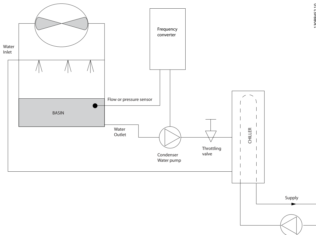
Afbeelding 2.20 De VLT-oplossing
