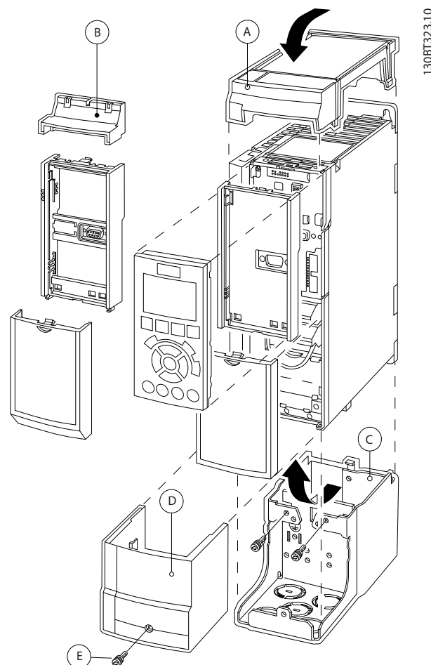
Afbeelding 3.19 Behuizingstype A2
