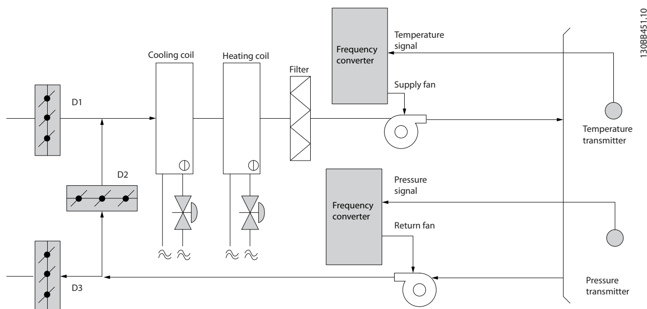
Afbeelding 2.18 De VLT-oplossing
