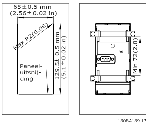
Afbeelding 3.18 Afmetingen
