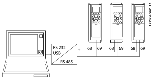
Afbeelding 8.1 Parallelle aansluitingen
