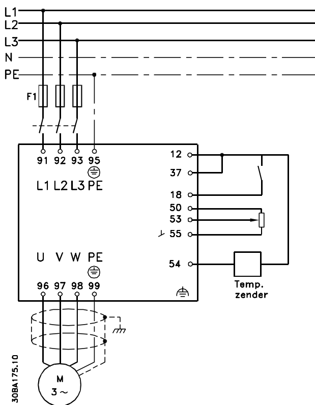
Afbeelding 2.31 Voorbeeld van PID-regeling met terugkoppeling
