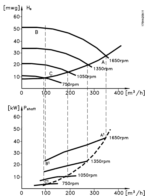
Afbeelding 2.13 Voorbeeld met wisselende stroming
