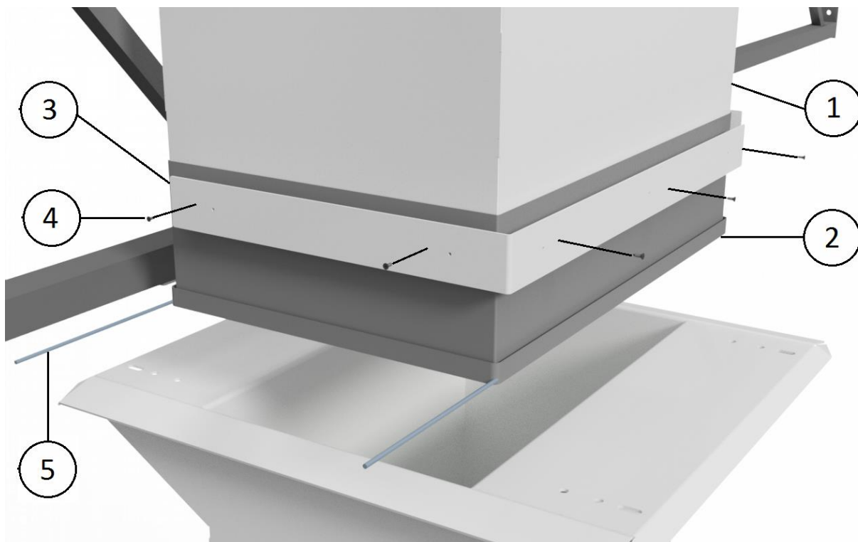
Figuur 10 Montage tussenstuk
