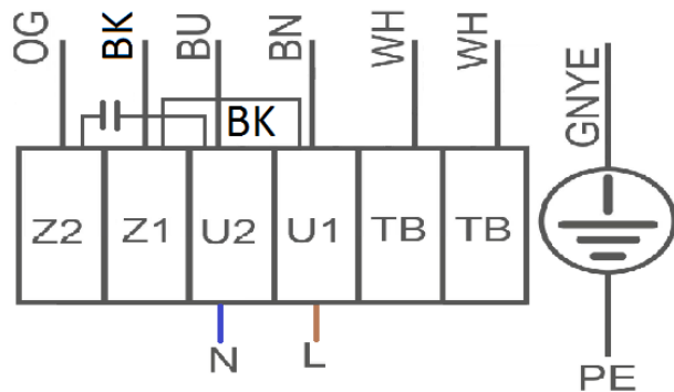
Figuur 24 Aansluitschema ZN045 AC
