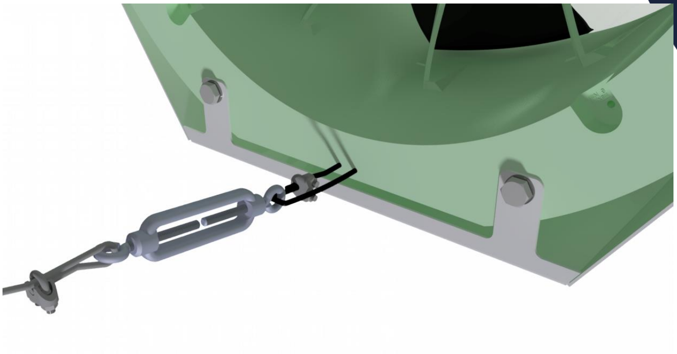
Figuur 7: Bevestiging spanwartel aan ventilator
