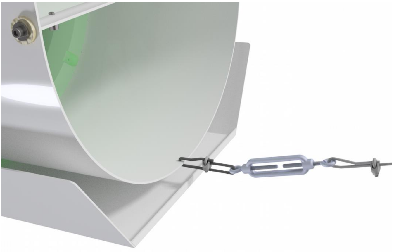
Figuur 8 Bevestiging spanwartel aan Airmix behuizing
