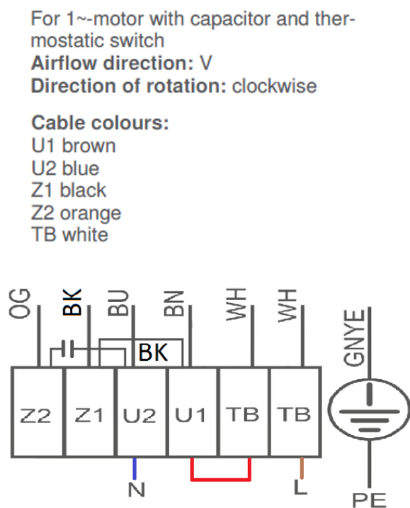
Figuur 22 Aansluitschema
