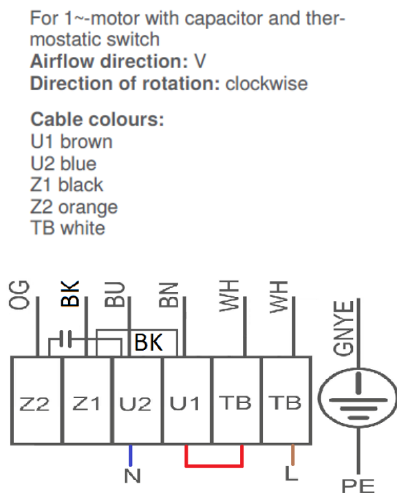
Figuur 17 Aansluitschema
