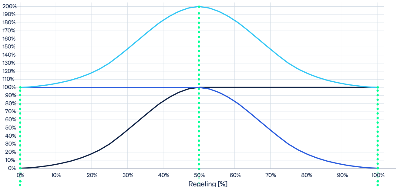
Debietkarakteristiek mengklep - 200% regeling
