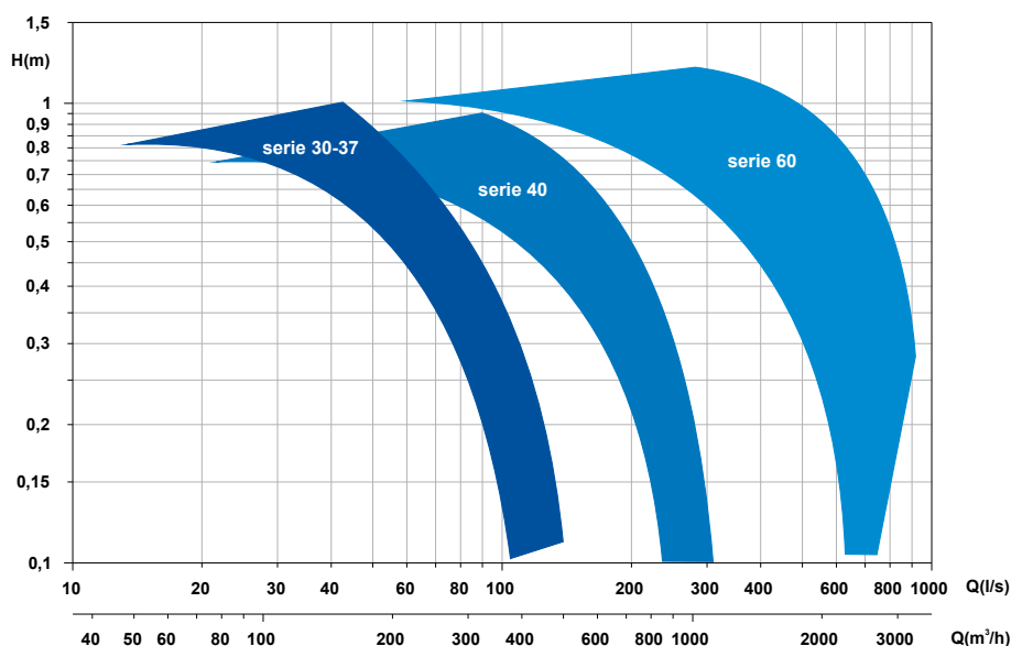
Capaciteitengrafiek N serie 50 HZ
