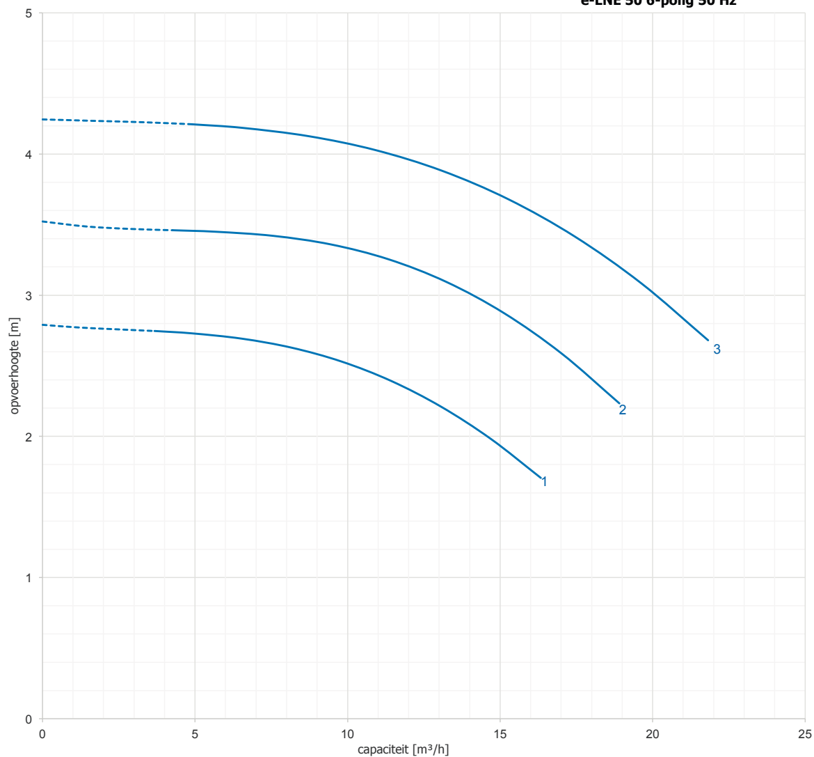
e-LNE 50 6-polig 50 Hz
