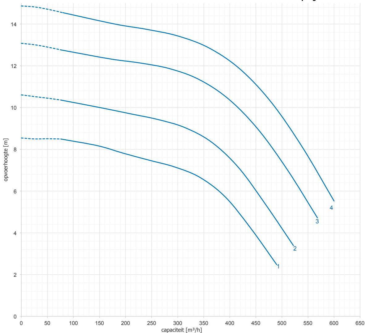
e-LNE 250 6-polig 50 Hz
