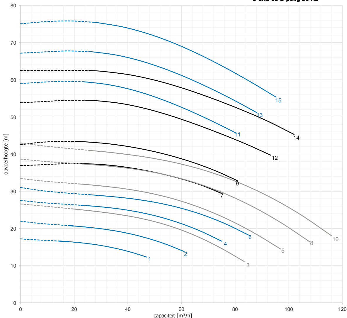
e-LNE 65 2-polig 50 Hz
