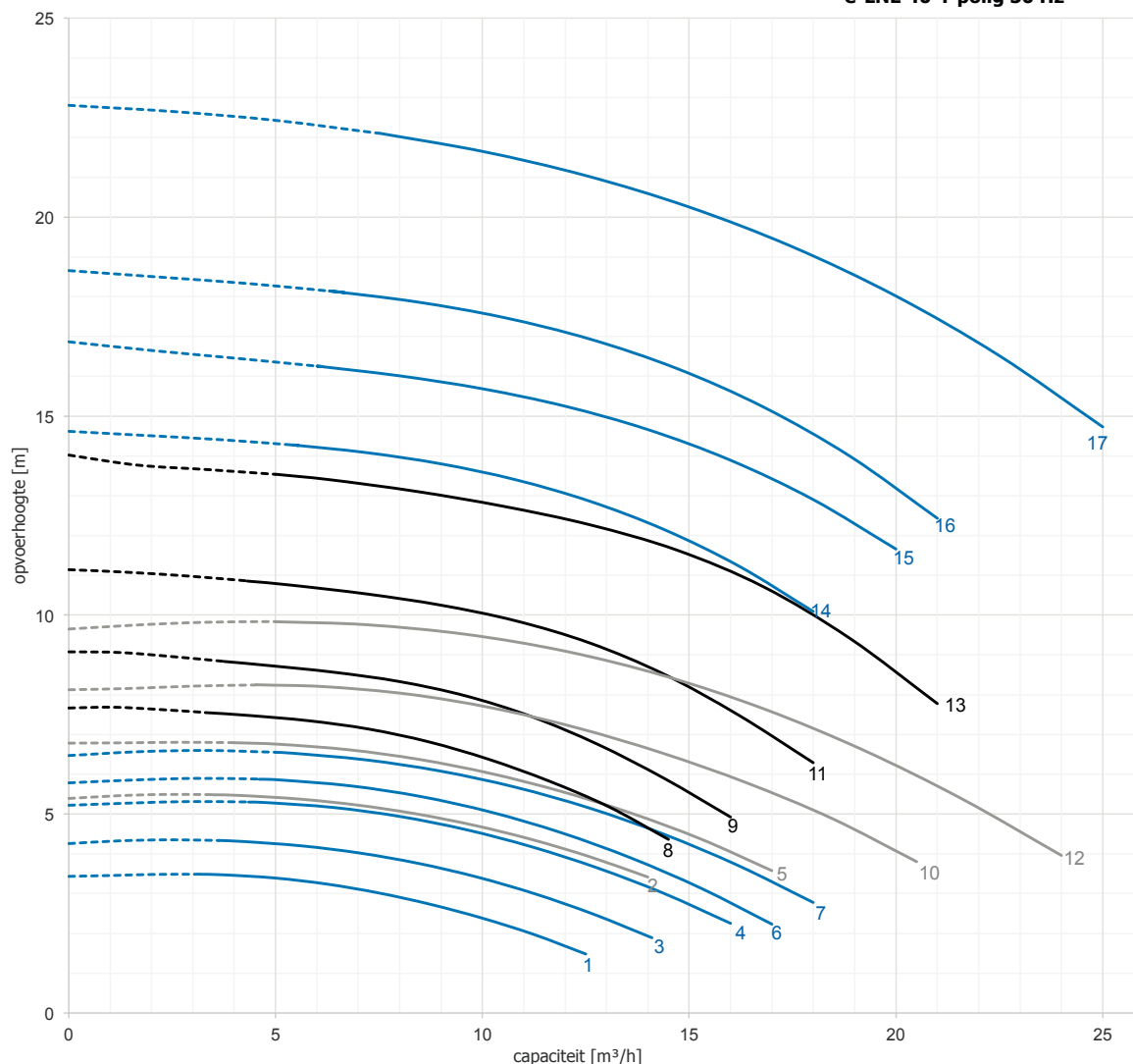
e-LNE 40 4-polig 50 Hz
