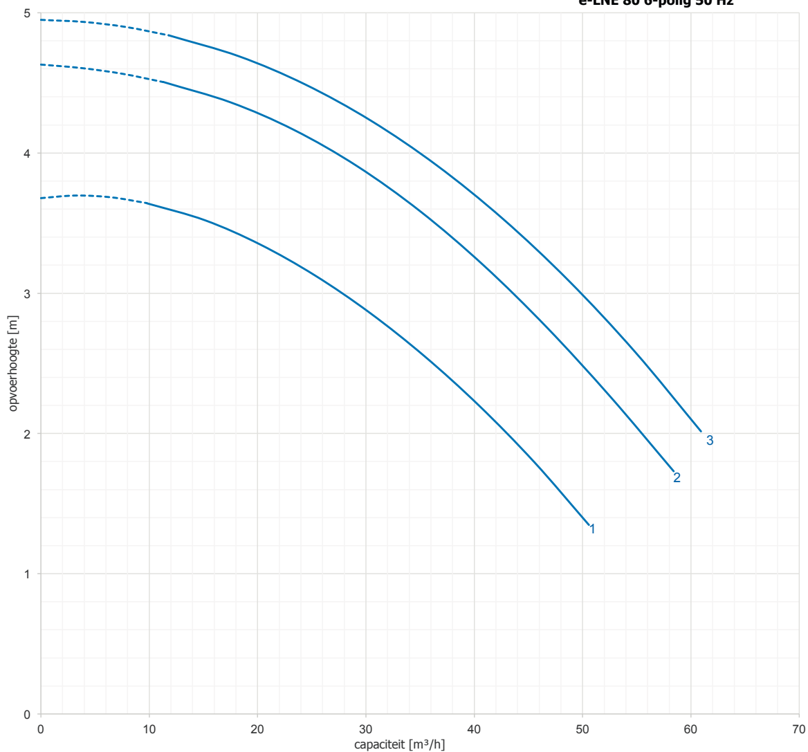
e-LNE 80 6-polig 50 Hz
