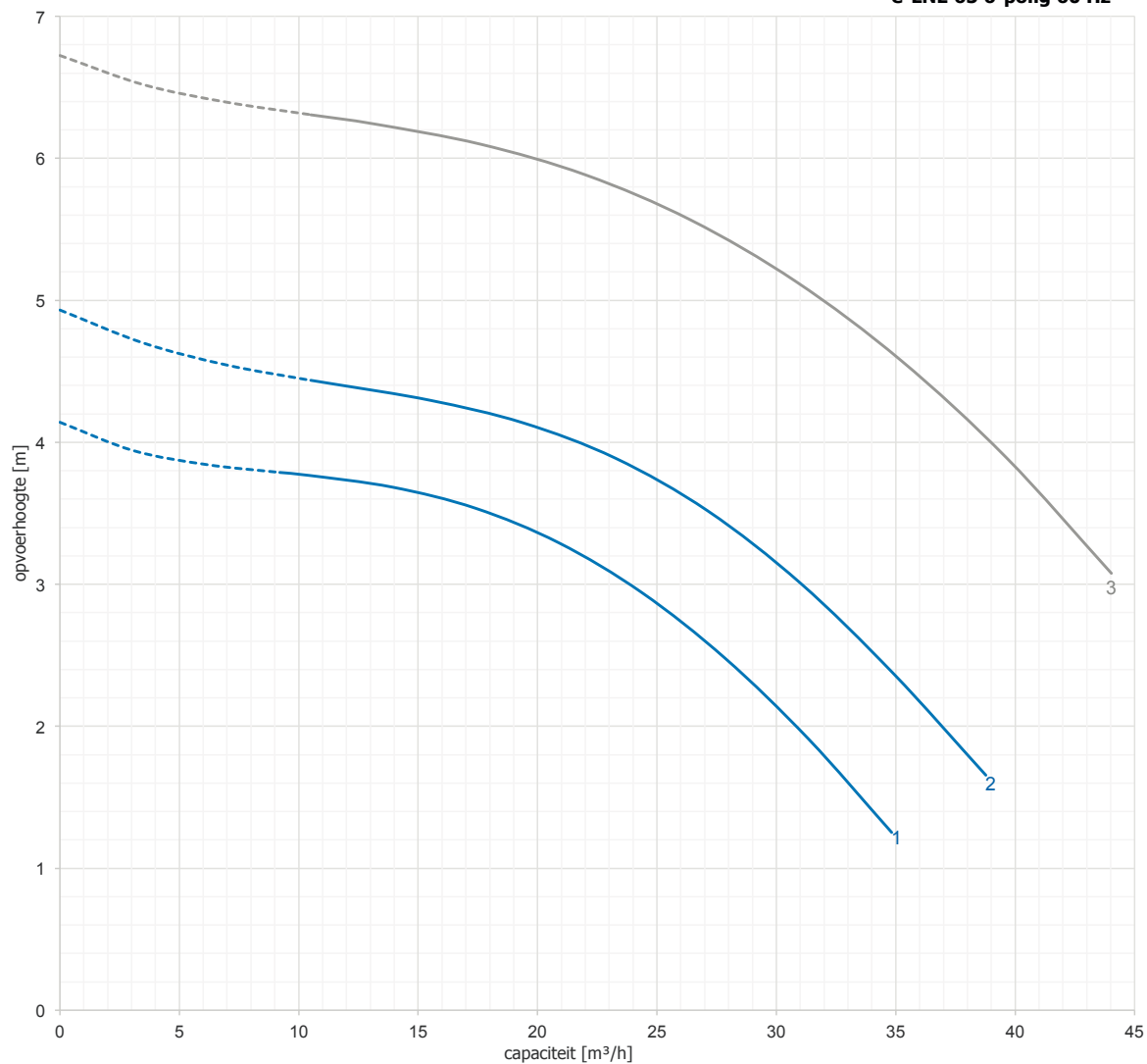
e-LNE 65 6-polig 60 Hz
