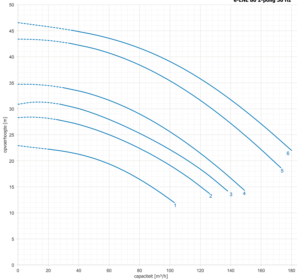
e-LNE 80 2-polig 50 Hz
