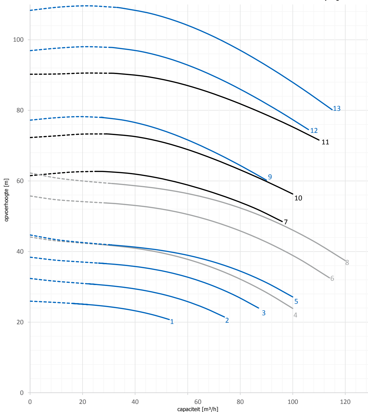
e-LNE 65 2-polig 60 Hz
