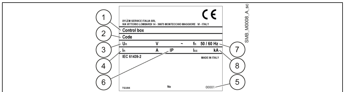
Afbeelding 4: Gegevensplaatje van de schakelkast
