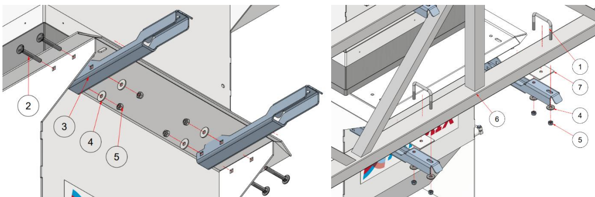
Figuur 4 Montage Airmix m.b.v. de verlengde ophangbeugel set
