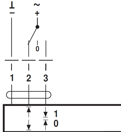
Figuur 30 klepaandrijving aansluitschema
