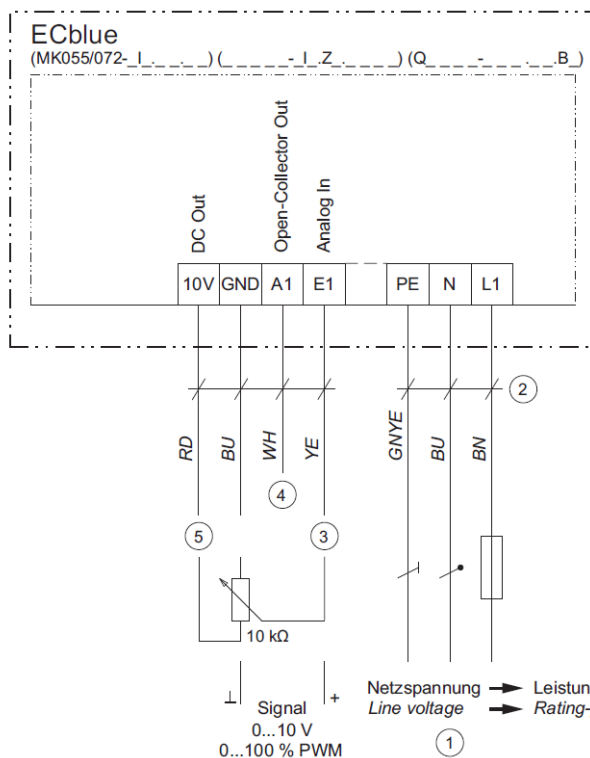
Figuur 27 (links) Aansluitschema ZG045 EC-ventilator
