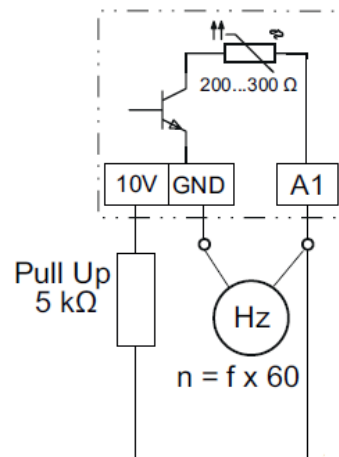
Figuur 27 (links) Aansluitschema ZG045 EC-ventilator
