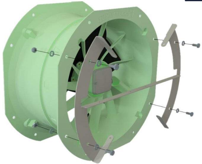
Figuur 17 Montage bevestigingsbeugel
