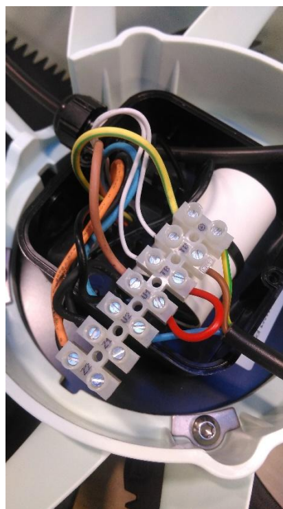
Figuur 23 Aansluiten Thermisch contact
