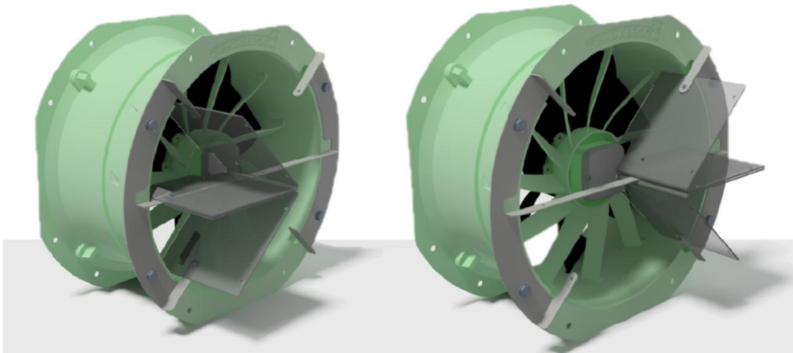
Figuur 16 Extra neer- (links) of opwaartse (rechts) restrictie van de luchtstroom
