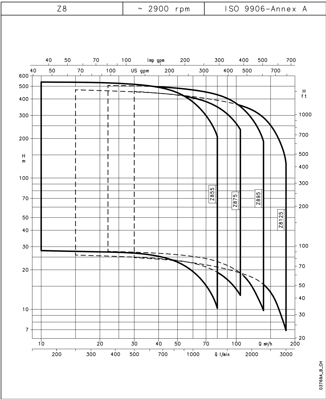
Capaciteitengrafiek Z8 serie bij 50 Hz, 2-polig
