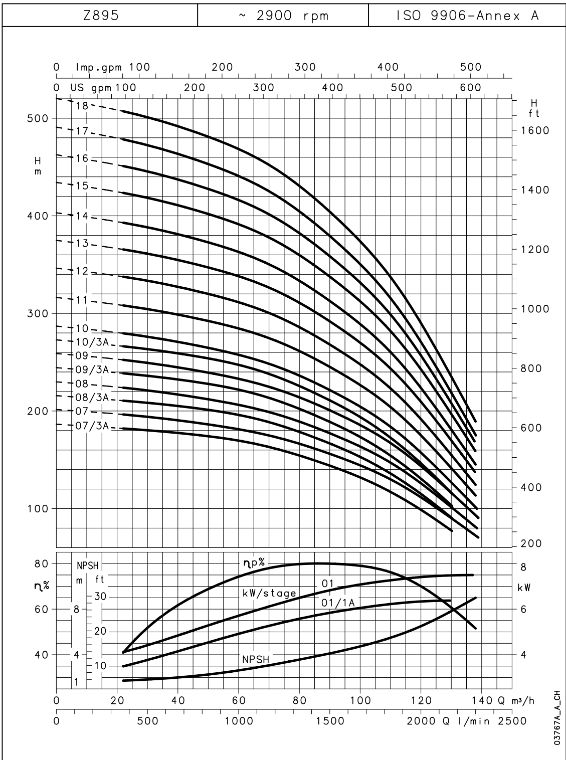
Capaciteitengrafiek Z895 serie 7-18 waaiers bij 50 Hz, 2-polig
