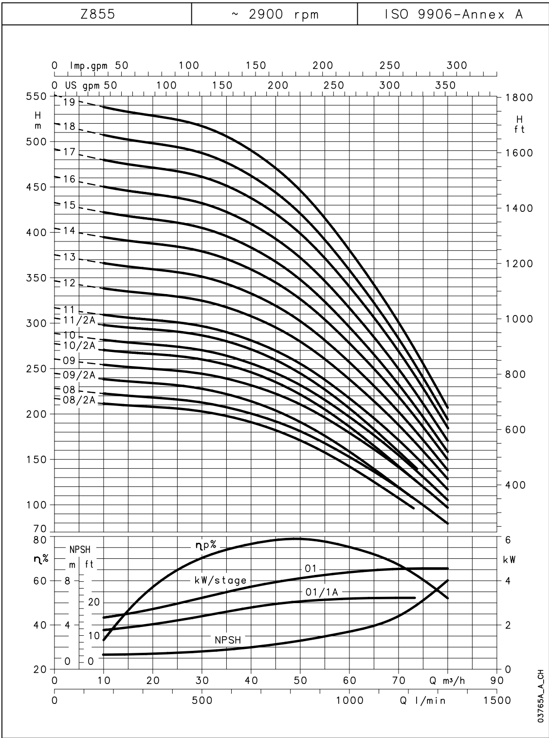
Capaciteitengrafiek Z855 serie 8-19 waaiers bij 50 Hz, 2-polig
