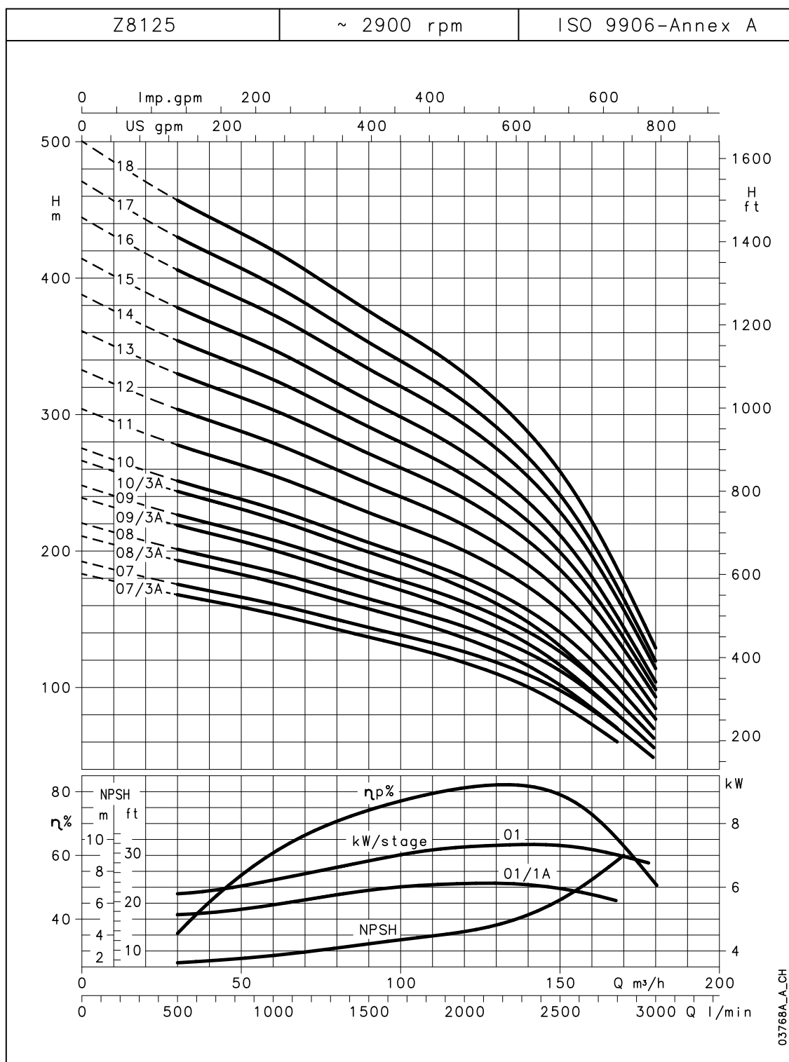
Capaciteitengrafiek Z8125 serie 7-18 waaiers bij 50 Hz, 2-polig
