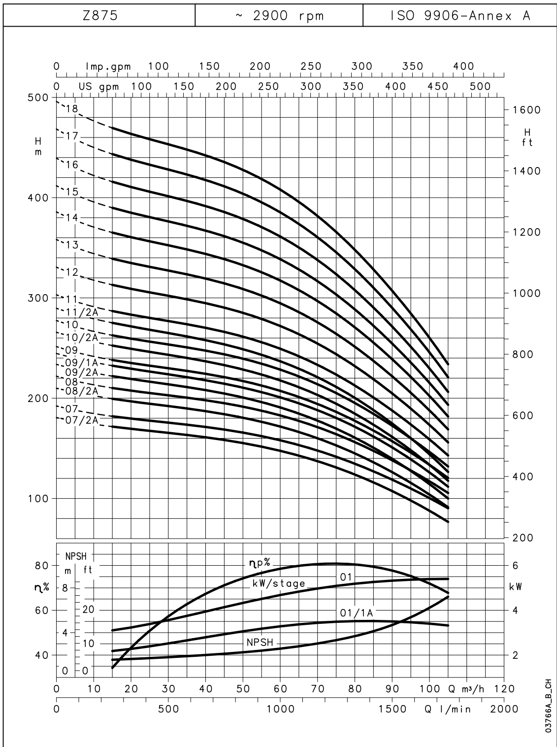
Capaciteitengrafiek Z875 serie 7-18 waaiers bij 50 Hz, 2-polig
