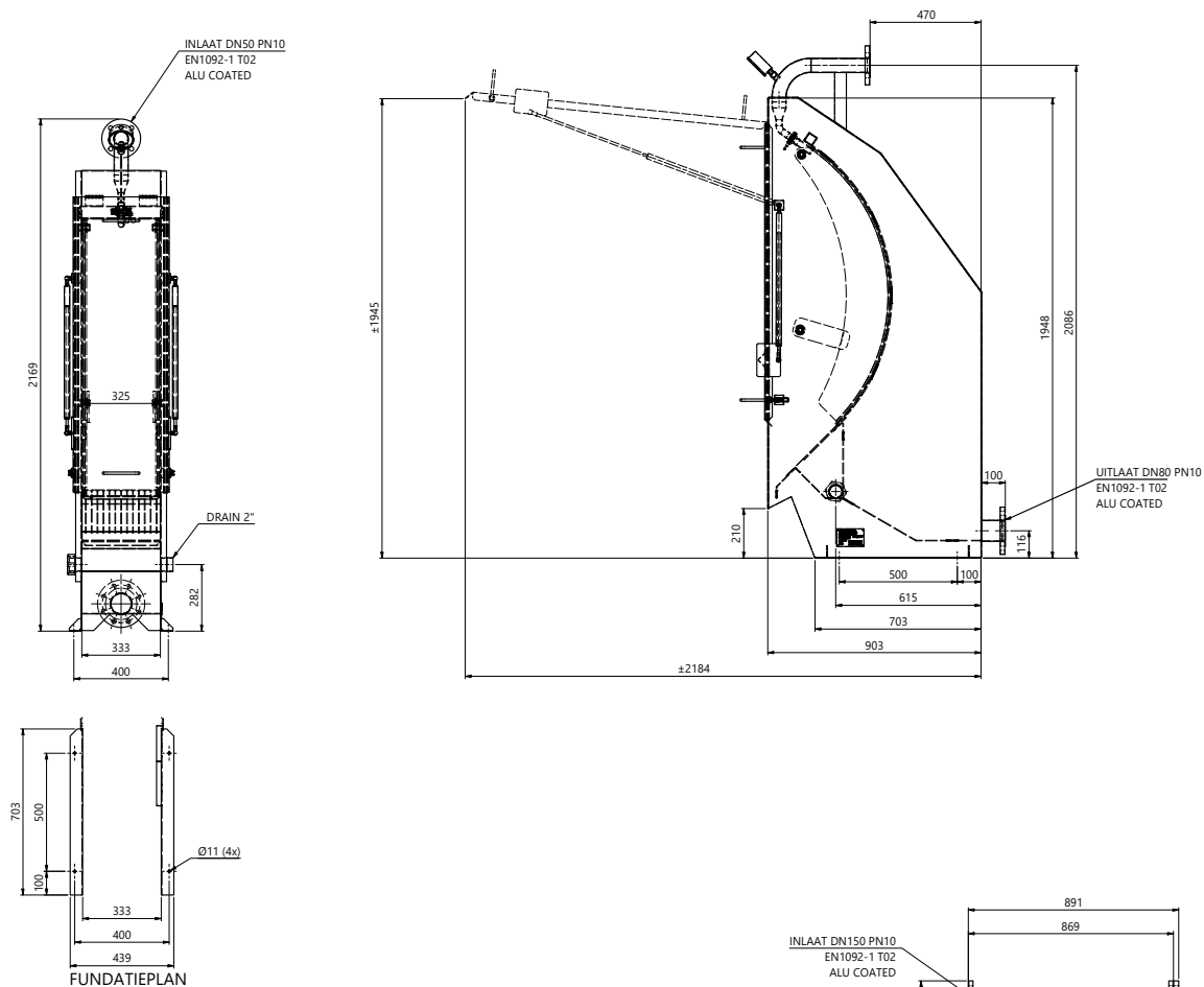
Tekening zeefbocht 300DT
