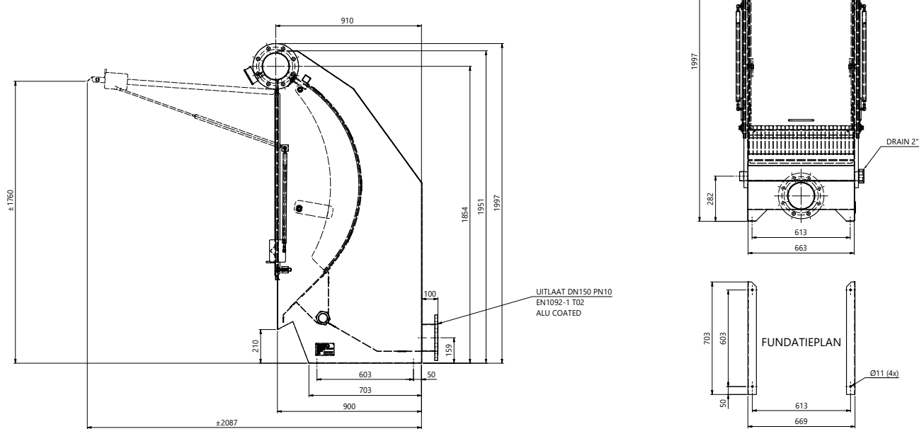
Tekening zeefbocht 600DT
